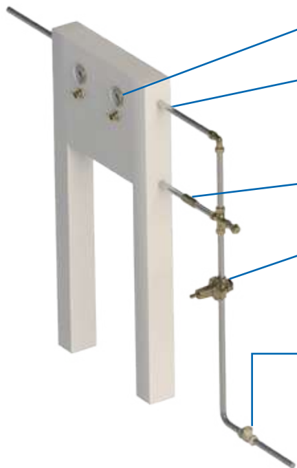
Коллектор среднего и низкого давления и нагнетательные системы
